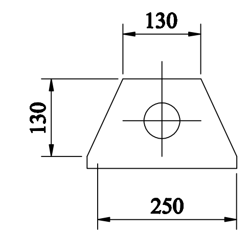
LIFT LUG
